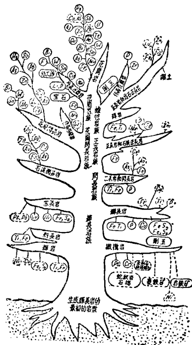
圖 2. 與火成岩類有關的元素及礦物分布圖
