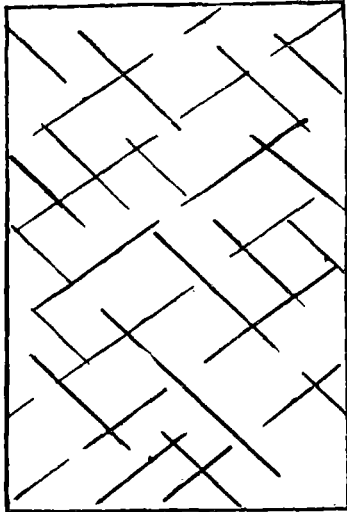
圖 1. 鈦鉄礦（黑色条帶）沿磁鉄礦（圖底）八面体%理填充之格狀結構
