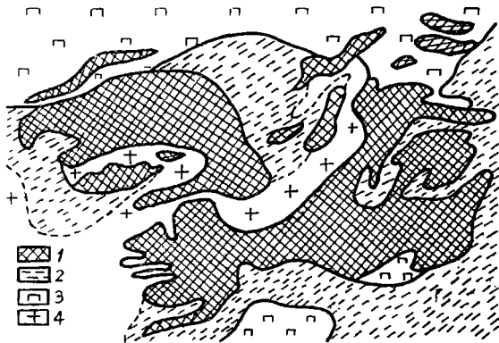
圖 3. ×× 号礦体地表地質平面略圖 1—礦体；2—一片輝狀輝長岩；3—斜長岩；4—輝長岩
