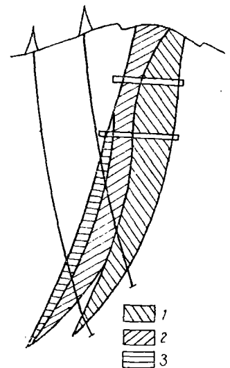
圖4. 1—I級品礦石；2—II級品礦石；3—III級品礦石
