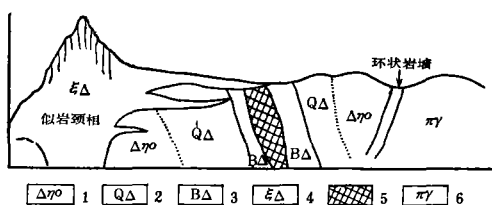
图3 龙潭含矿角砾岩体各类角砾岩分布示意图
