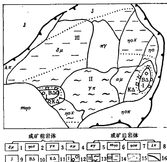
图4 大庄科钼矿床蚀变类型及分带示意图
