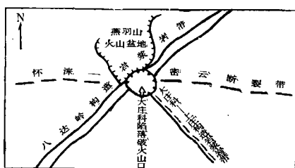
图1 大庄科陷落破火山口构造位置简图
