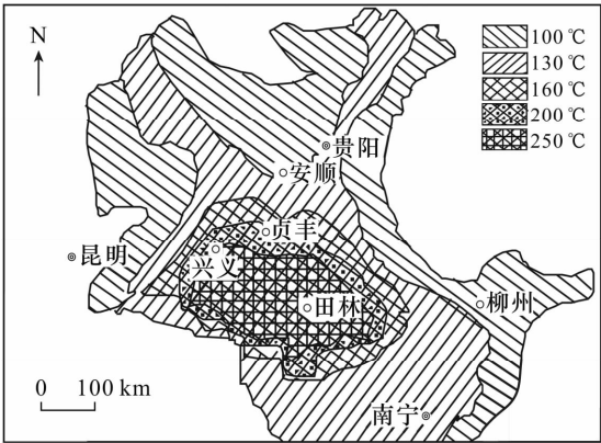
图 3 滇黔桂地区上二叠统古地温分布图 [10] Fig.3 Distribution of Upper Permian paleo-geotemperatures in Yunnan-Guizhou-Guangxi area [10]
