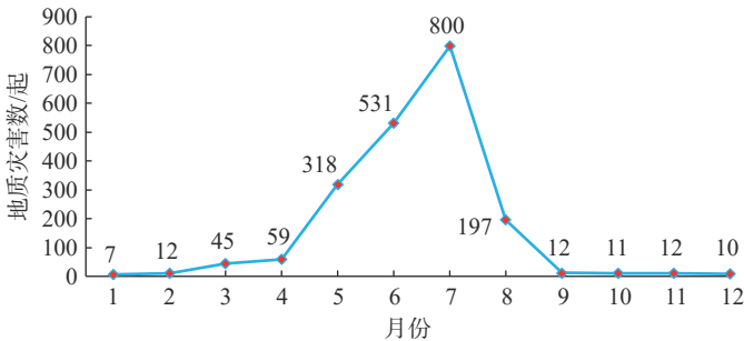
图 2 2012—2021 年月均地质灾害发生数量
