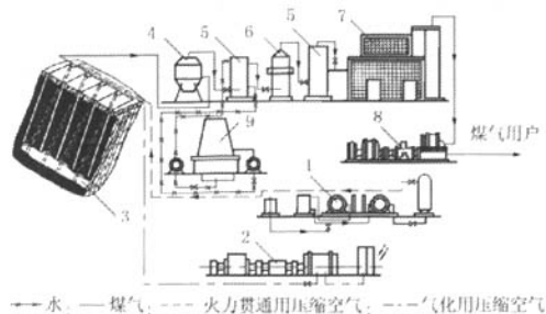
图1 地下气化站工艺流程图
