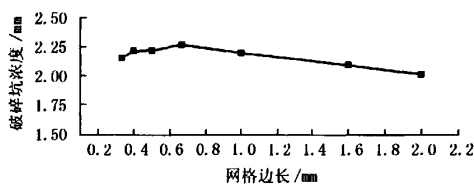
图9 混凝土板的破碎坑深度(不同网格边长)
