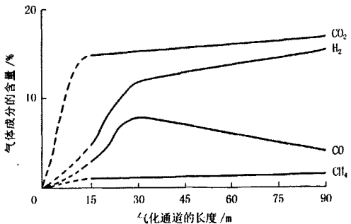
图 6 煤气成分与气化通道长度的关系曲线
