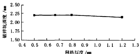
图10 混凝土板的破碎坑深度(不同网格厚度)
