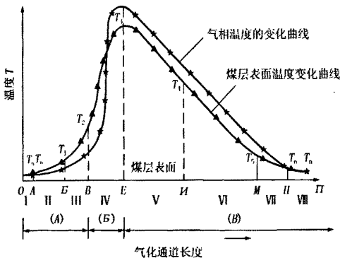
图 4 温度变化特性与煤层表面分区关系示意图 OA —进气区; AB —进气干燥区; BB —燃烧准备区; BE —放热反应区; EH —吸热反应区; HM —热分解区; MH —煤气干燥区; HI —煤气区
