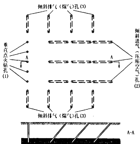
图9 安格连煤田平缓水平厚煤层条件下地下气化施工示意图
