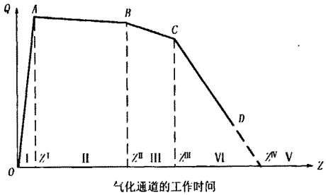
图 5 气化通道内气体燃烧热量 Q 与工作时间的关系
