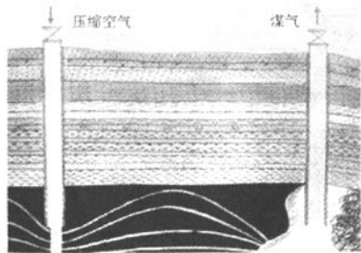
图7 渗透式火力贯通示意图
