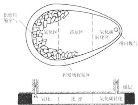
图2 煤炭地下气化过程示意图
