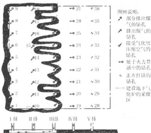
图8 莫斯科郊外地下气化站采用的煤炭气化示意图
