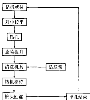
图2 旋喷桩施工流程图
