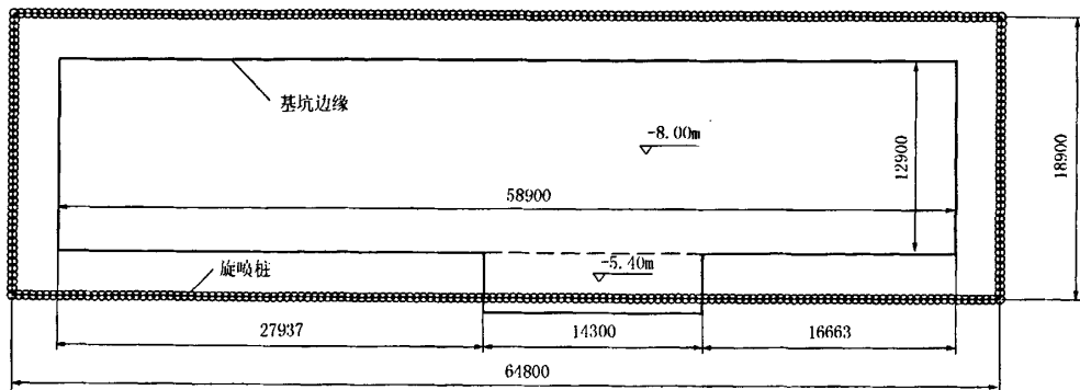
图1 单排旋喷桩止水帷幕布置图
