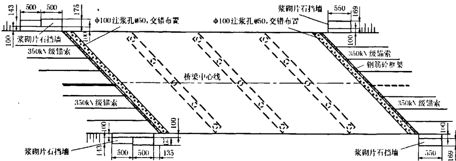
图 2 注浆孔布置平面图
