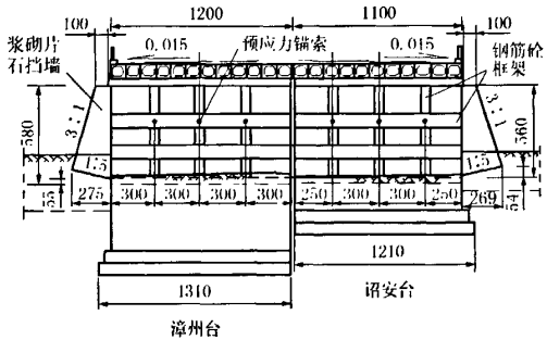
图4 预应力锚索设置示意图
