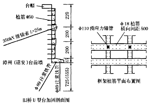
图3 注浆孔布置剖面图
