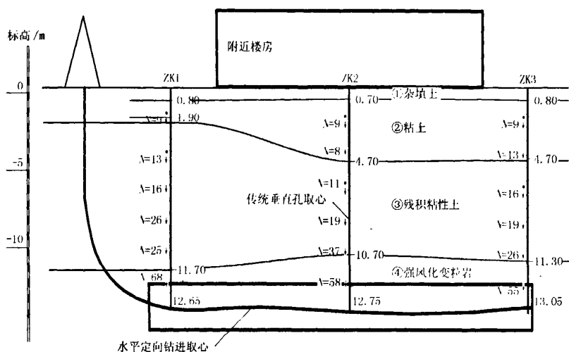
图3 选址点上部建筑物与勘探点工程地质剖面图
