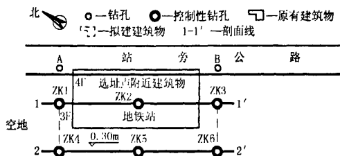
图 2 选址点附近建筑物与勘探点平面位置图
