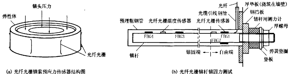
图 4 武汉理工大学进行的光纤锚固力测试
