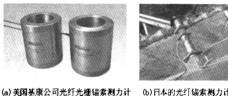
图 3 国外的光纤锚索测力计
