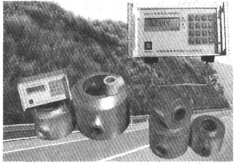
(a) 锚索测力计及BMS-2型便携式读数仪
