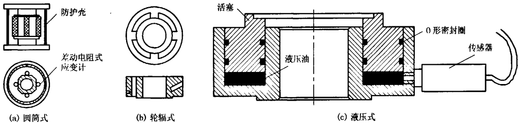
图1 锚索预应力传感器结构示意图
