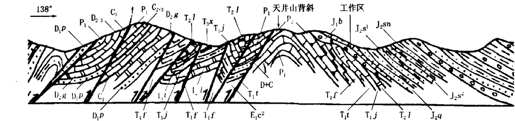
图 1 区域构造形式剖面图
