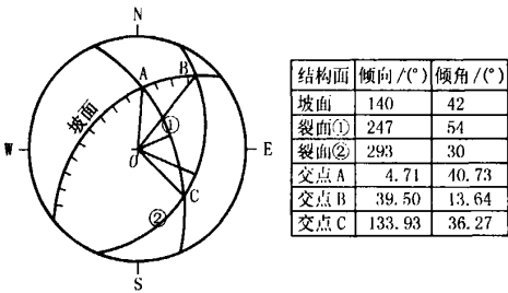
图 2 基岩节理赤平投影图
