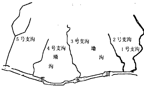
图5 研究区堆积体地表水系发育特征图
