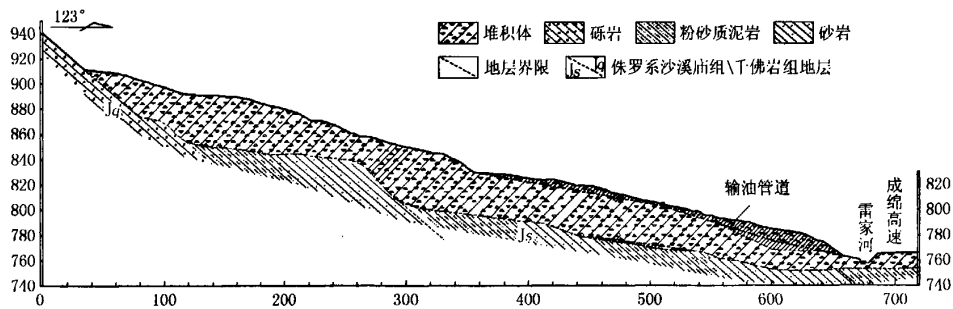
图 4 前扇形段斜坡纵剖面图
