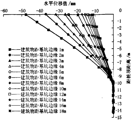
图2 围护桩水平位移随建筑物位置变化图
