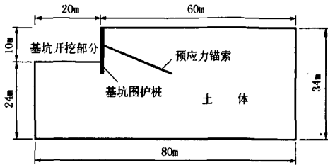
图1 基坑模型示意图
