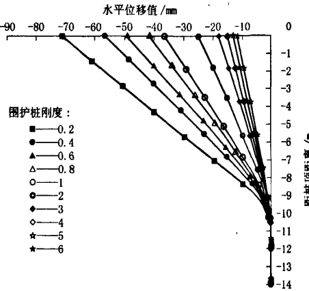
图3 围护桩水平位移随自身刚度变化图
