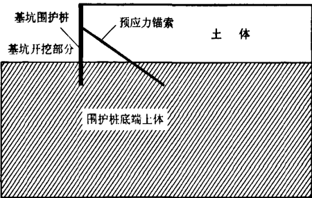
图 4 基坑围护桩底端土体示意图
