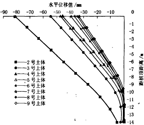
图 5 围护桩水平位移随围护桩底端土体变化图
