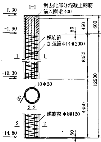
图3 围护钻孔灌注桩配筋图
