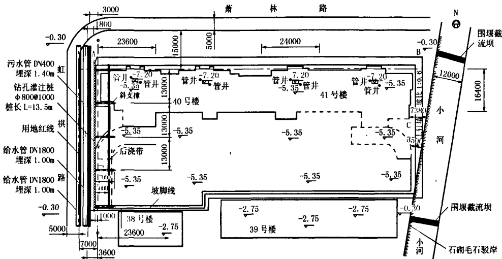
图 1 基坑平面布置图
