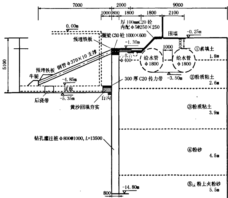
图 2 支护结构剖面
