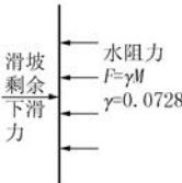
图 5 剩余下滑力和水阻力关系
