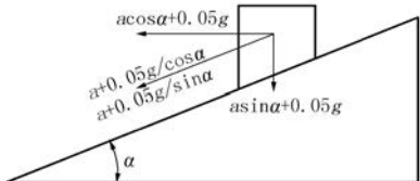
图 6 滑体下滑的受力分解图
