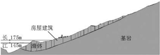
图 7 藕塘滑坡剖面及房屋建筑示意图
