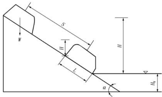
图 4 滑坡体涌浪预测各要素示意图
