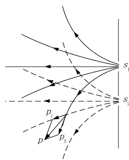
图 6 纵波干涉示意图
