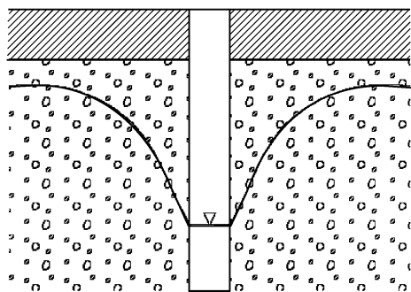
图 1 水泵洗井抽水漏斗示意图
