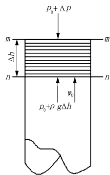
图 3 水锤压力导出示意图
