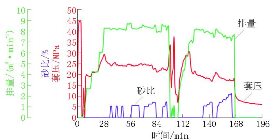
图 5 B32-3 井 4+5 号煤层压裂施工曲线
