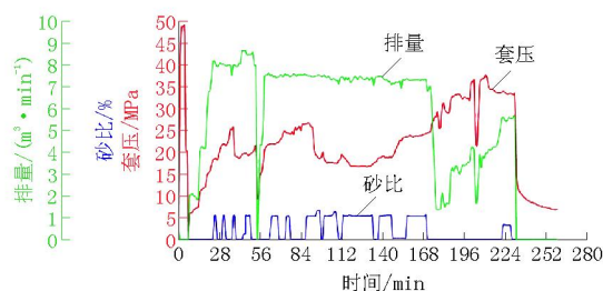
图2 B32-3井7+8+9号煤层压裂施工曲线
