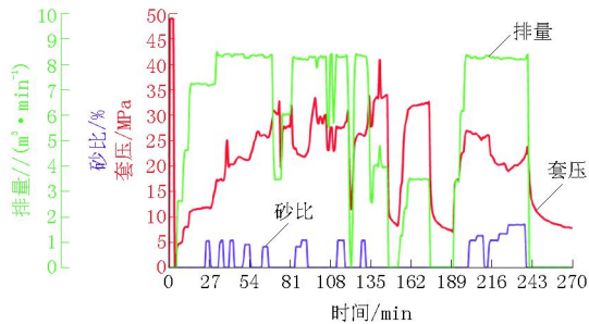
图8 B32-11井7+8+9号煤层压裂施工曲线
