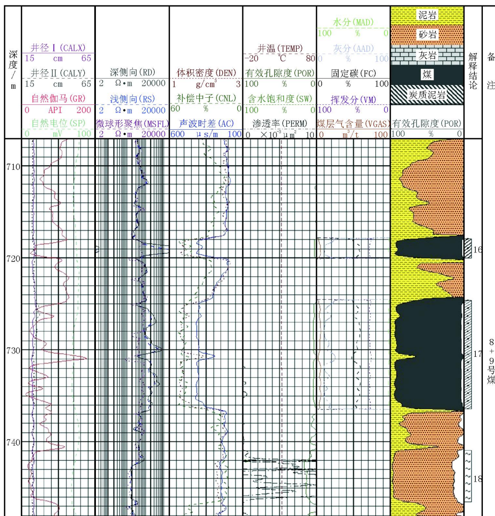
图3 B32-3井7+8+9号煤层的测井曲线
