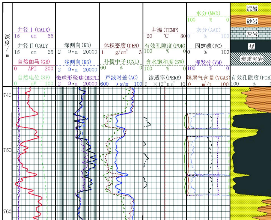
图6 B34-1井测井曲线解释
