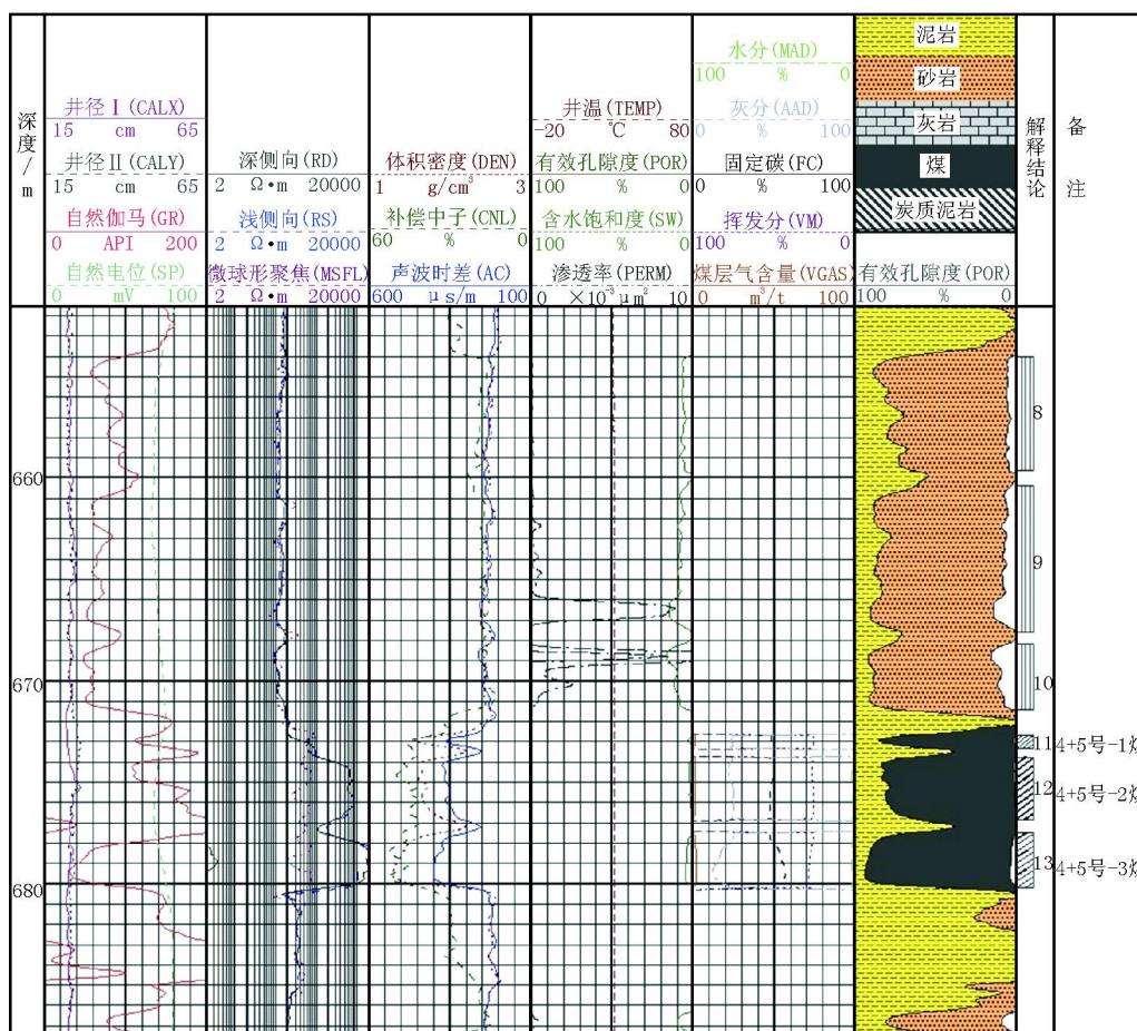
图 4 B32-3 井 4+5 号煤层测井曲线解释
