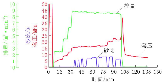
图7 B34-1井8+9号煤层压裂施工曲线
