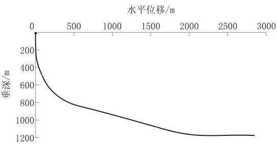
图 2 I38H 井垂直投影图
