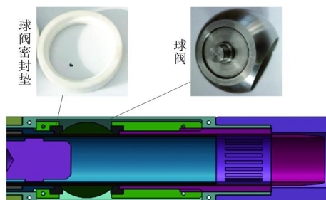
图3 球阀密封图
