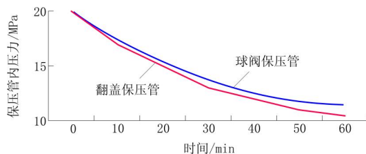
图6 球阀保压管和翻板保压管内压力随时间变化曲线
