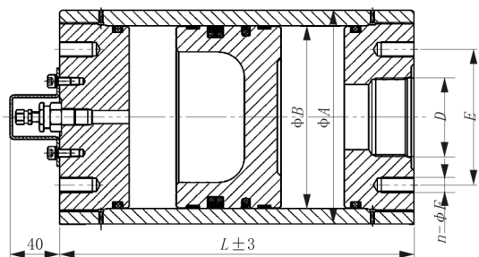
图2 活塞蓄能器简图
