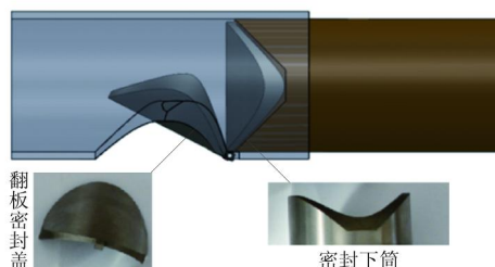
图4 单片翻板阀密封图
