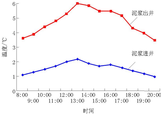
图4 泥浆制冷效果图
