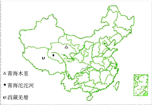
图 1 青藏高原陆域水合物勘探开发主要区域
