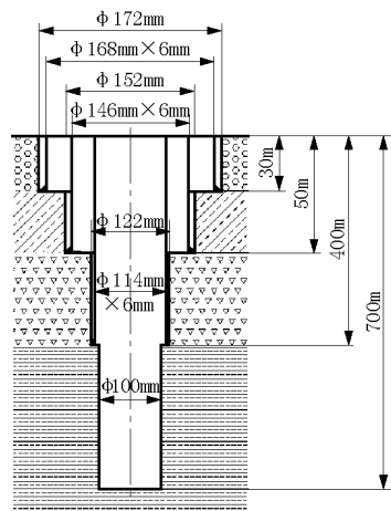
图 2 TK-2 孔钻孔结构图
