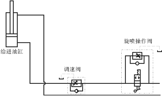
图 3 钻进回路工作原理
