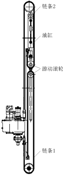
图 2 桅杆倍速机构
