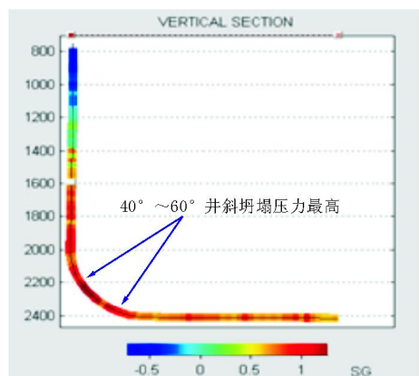
图 2 坍塌压力随井斜角的变化图
