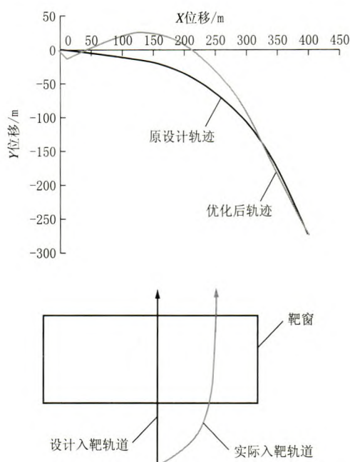
图 4 X2-9 井轨迹优化情况
