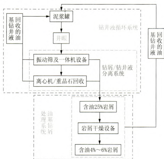
图6 钻井液回收示意图
