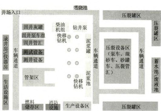
图 1 工厂化钻井作业布局图
