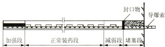
图2 预裂爆破装药结构示意图
