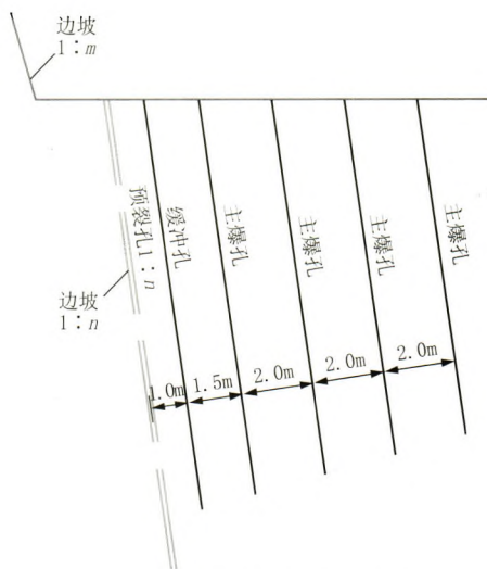
图3 预裂爆破钻孔剖面示意图
