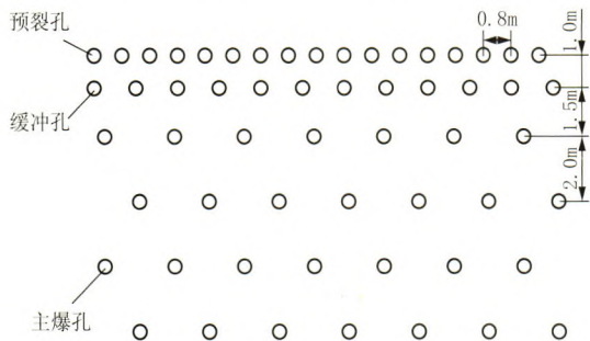
图1 布孔示意图
