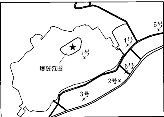
图 5 测点布置示意图
