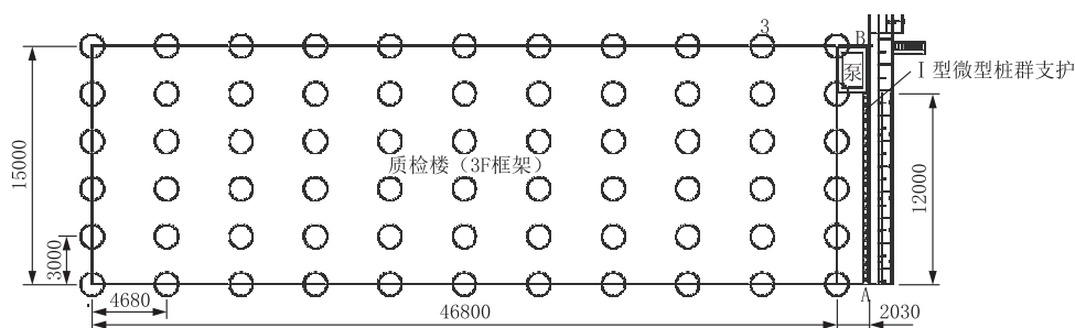
图3 静压桩位置布置平面示意
