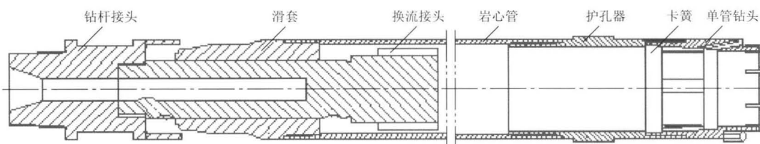
图 2 专用单管钻进取心工具
