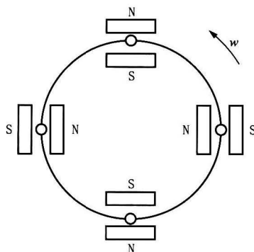
图5 钻头磁化(充磁、去磁)示意
