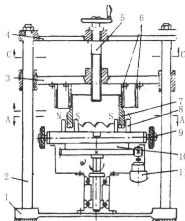
1—支座;2—导向杆;3—活动横梁;4—带螺杆的不动横梁;5—钻头给进螺杆;6—把钻头安装在试验台上用的带有螺纹的套;7—钻头;8—N和S磁铁;9—把磁铁移动到不同直径钻头用螺杆;10—转动的工作台;11—工作台驱动装置
