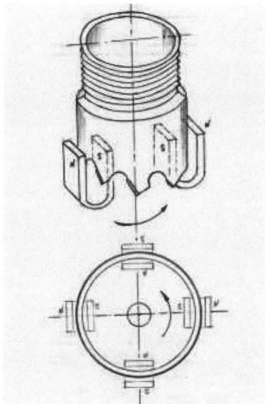
图7 在试验台上安装的钻头
