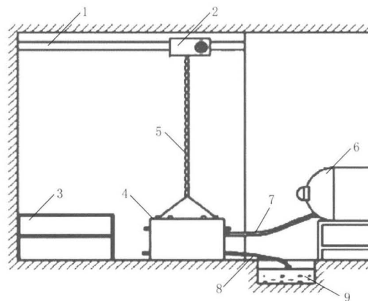
1—电葫芦横梁;2—电葫芦(提升装置);3—工作台;4—低温液态氮容器;5—链条;6—运输用液态氮罐 ИТК-5/0.25;7、8—压入隔热软管和放出隔热软管;9—放出池
