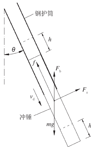
图1 冲锤下落受力示意
