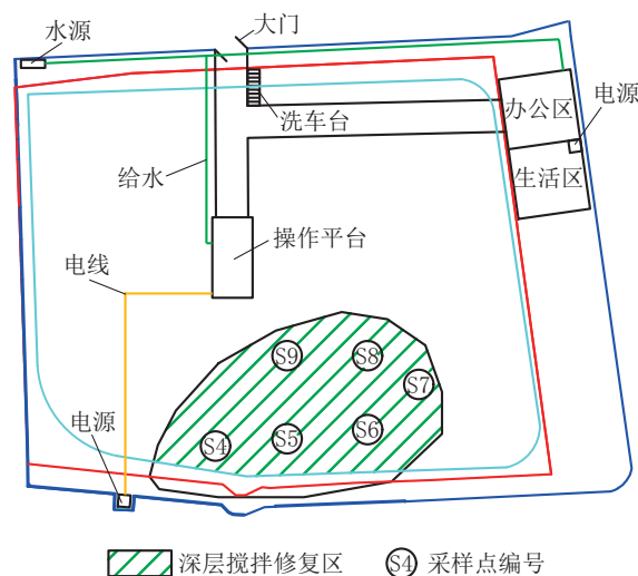
图2 自检采样点位平面布置
